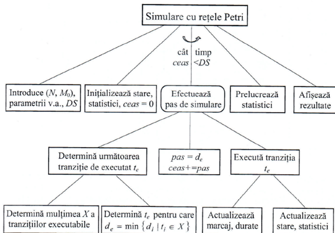
Fig. 4.10 – Structura algoritmului de simulare cu rețele Petri.
